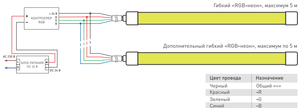
Схема 1. Подключение «гибкого неона»
